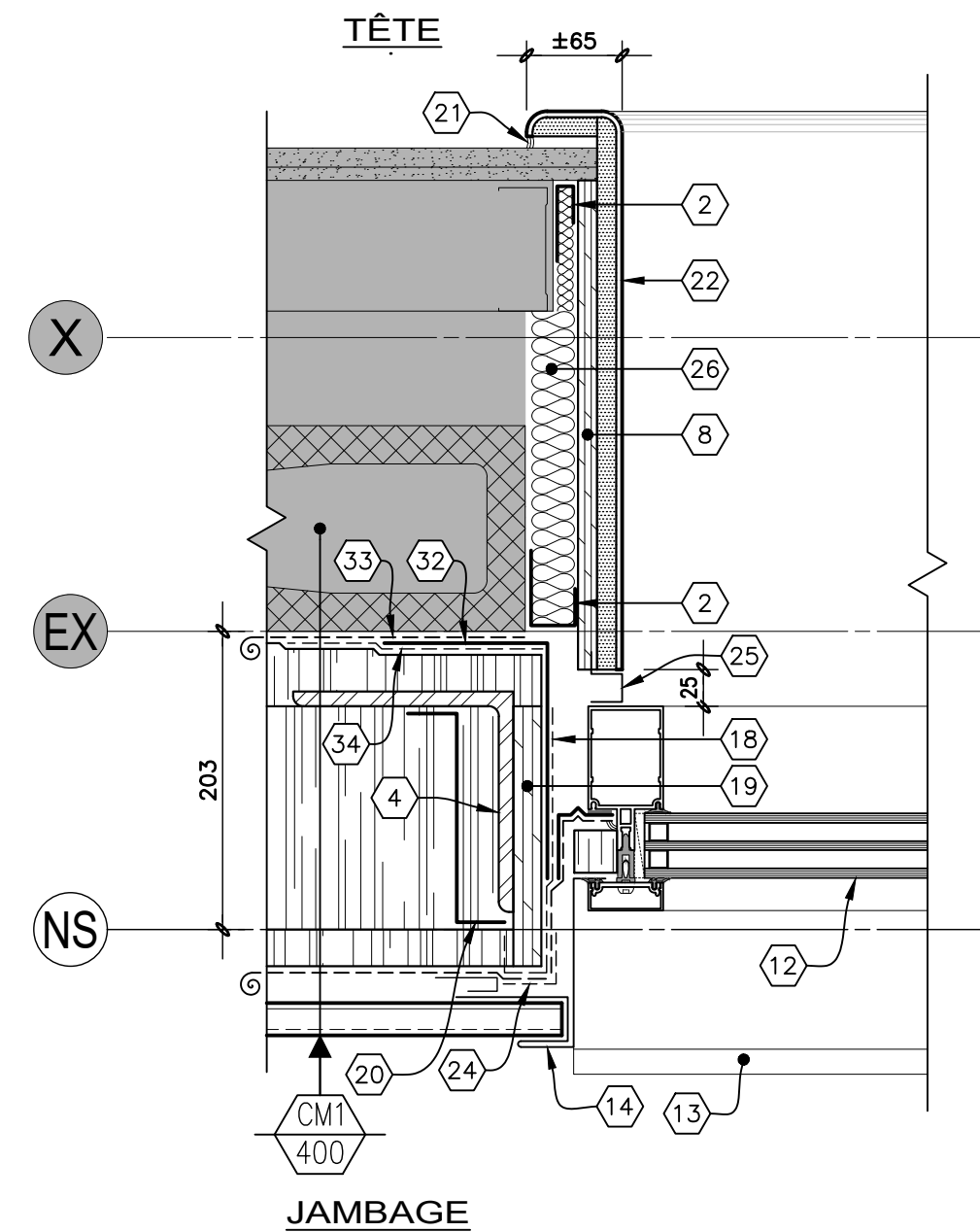
JAMBAGE
