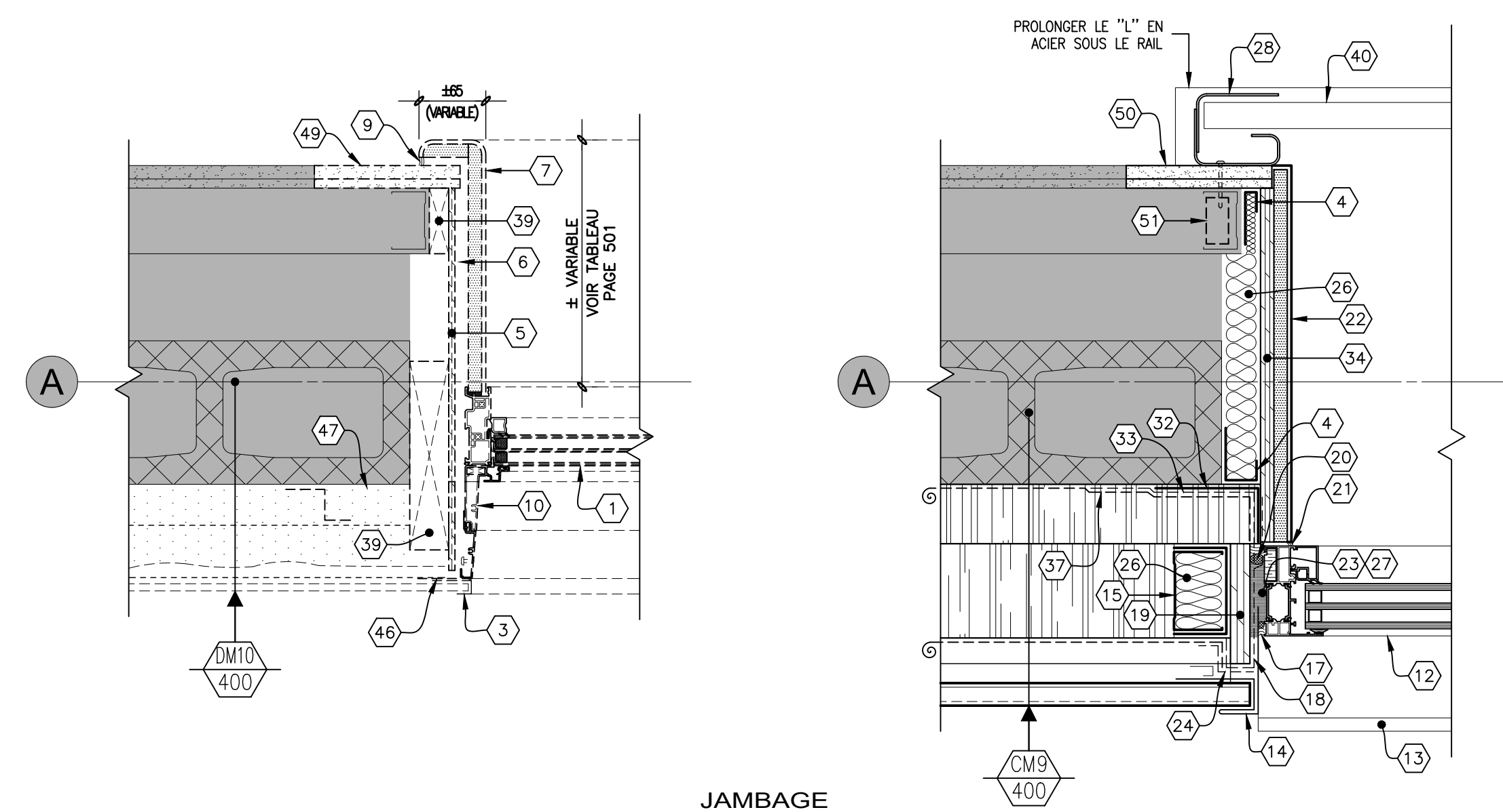
JAMBAGE
