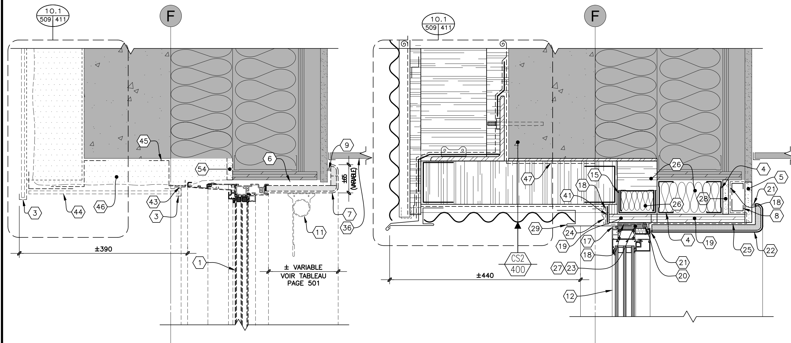
TÊTE
