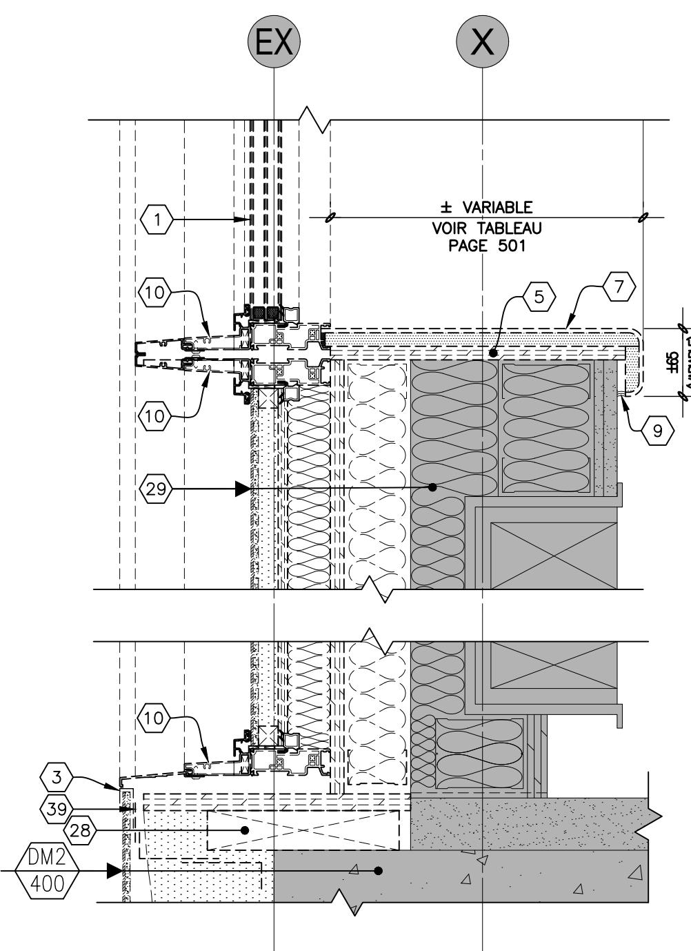
DÉMOLITION
