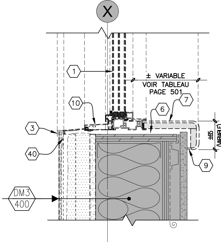
ALLÈGE
