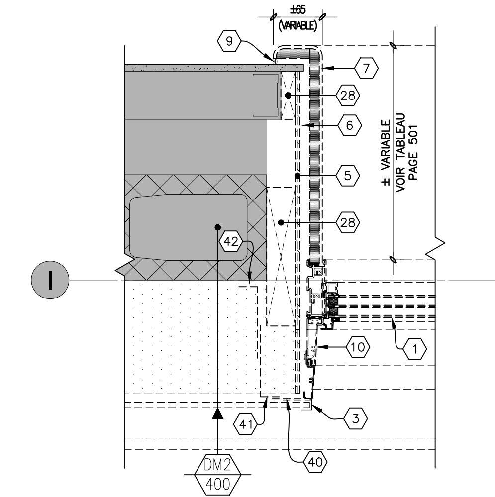
JAMBAGE
