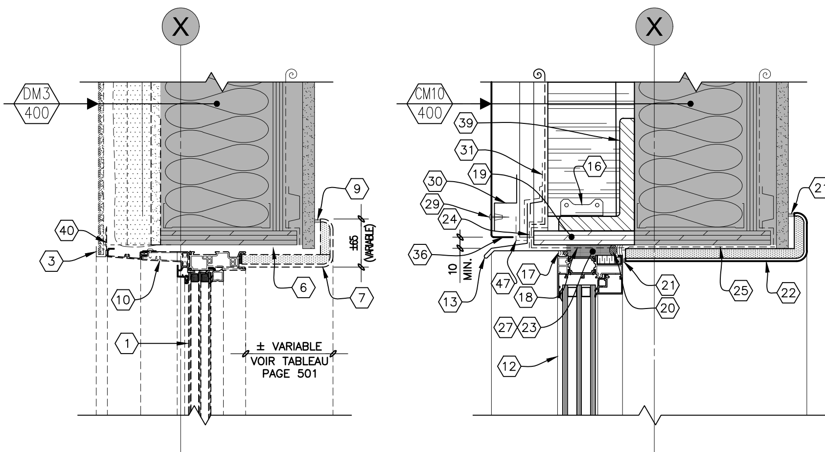
TÊTE
