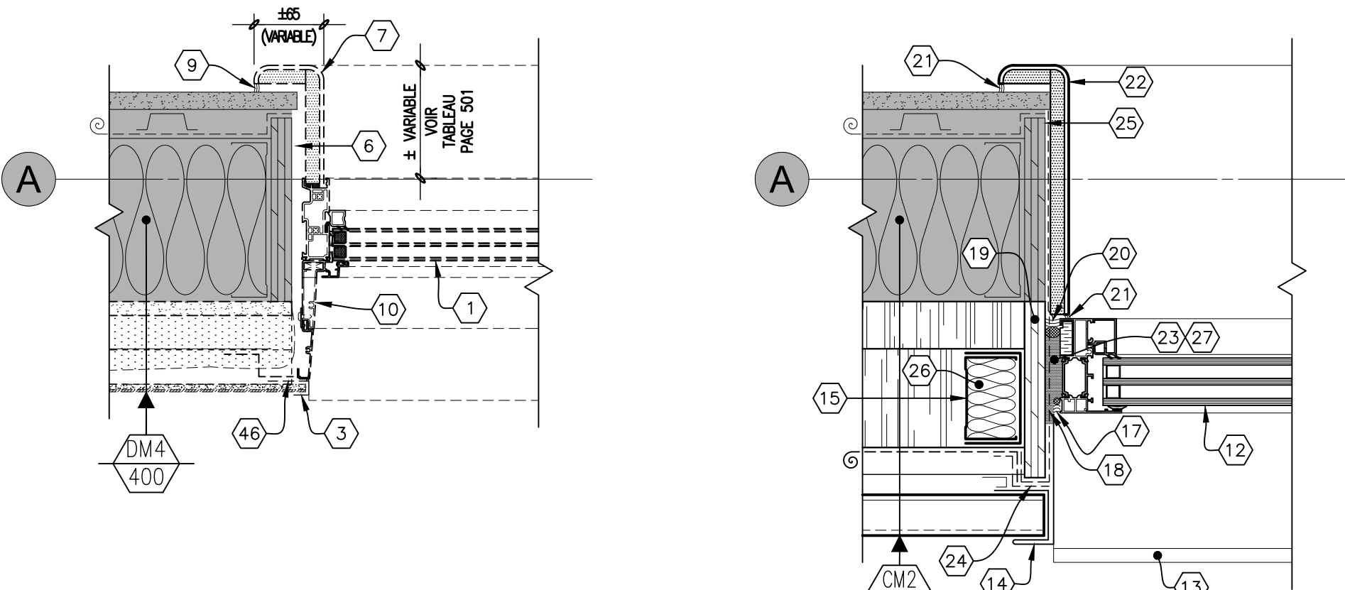
JAMBAGE
