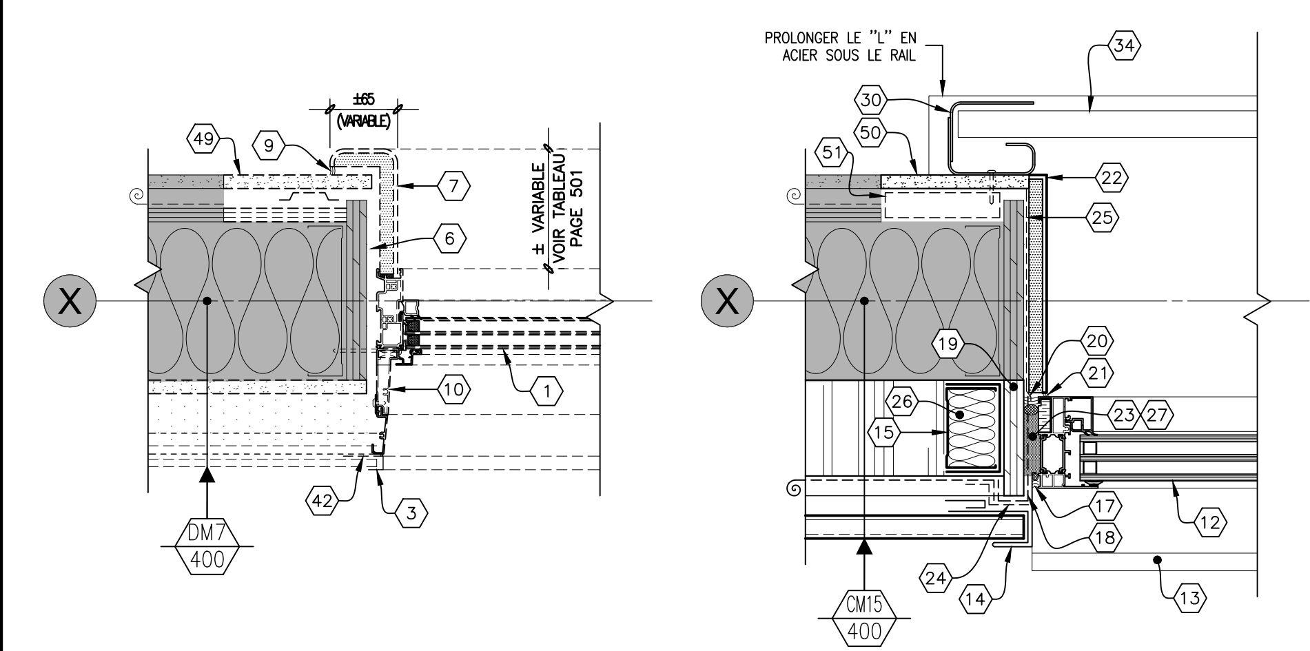
JAMBAGE
