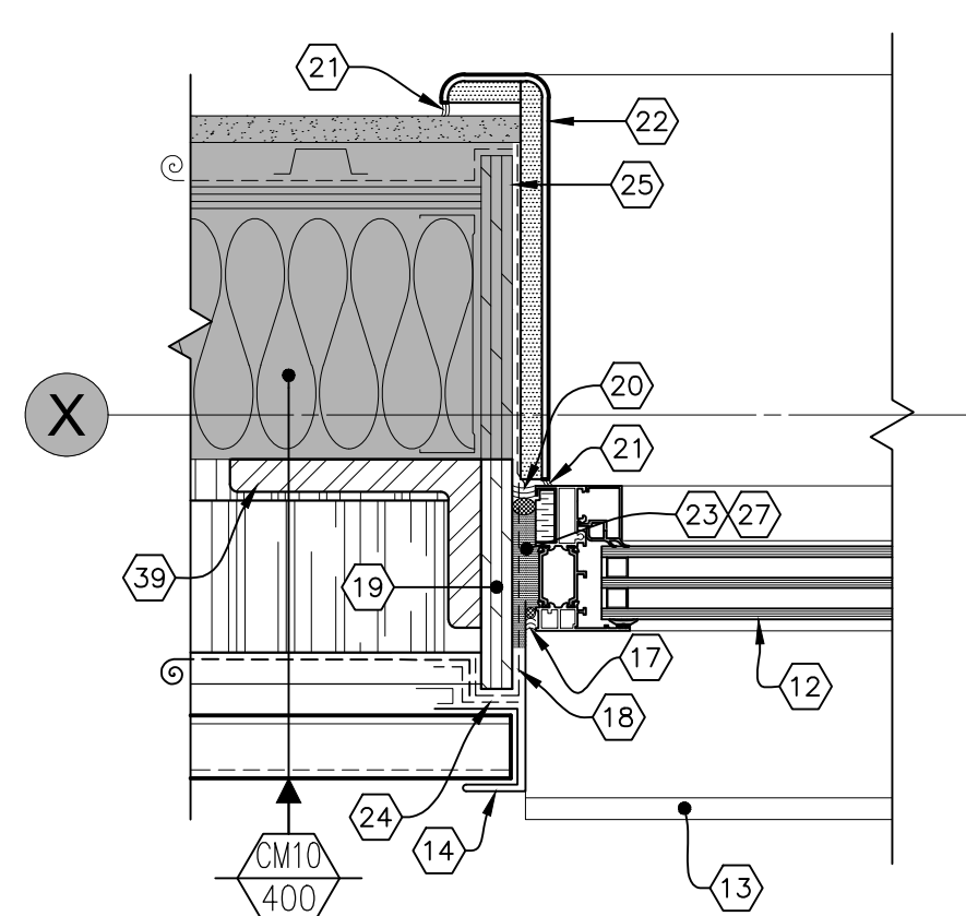
JAMBAGE
