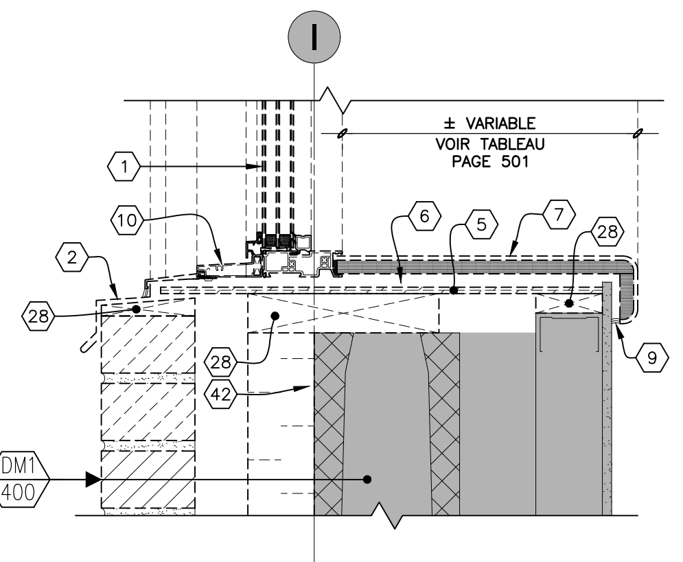
DÉMOLITION
