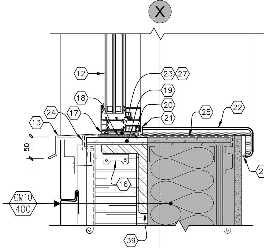
ALLÈGE
