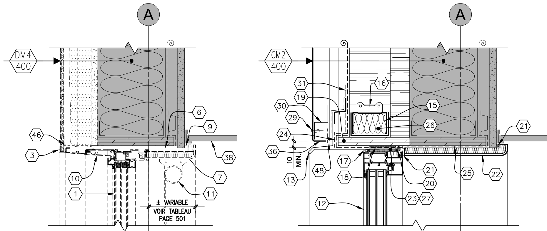
TÊTE
