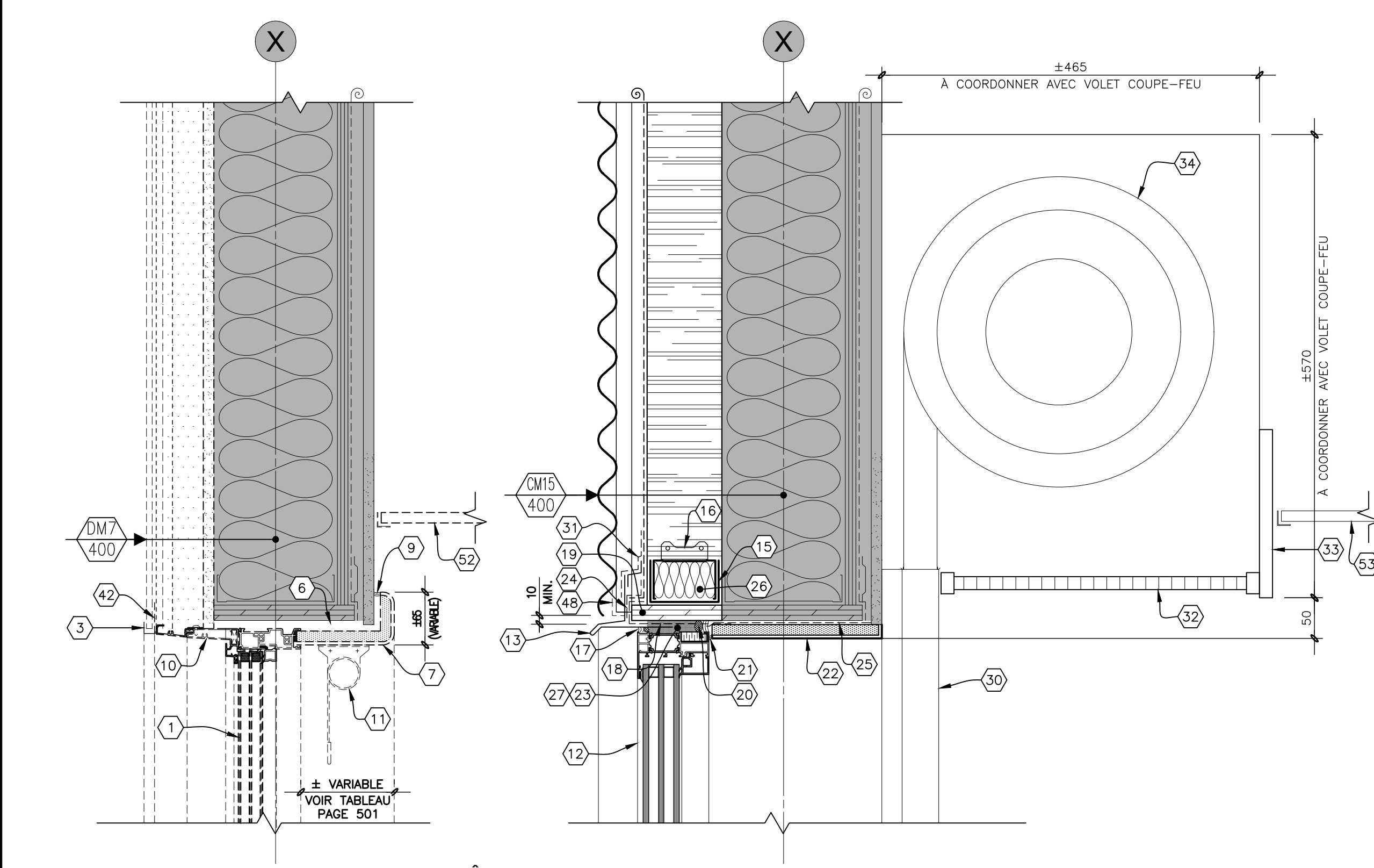
TÊTE
